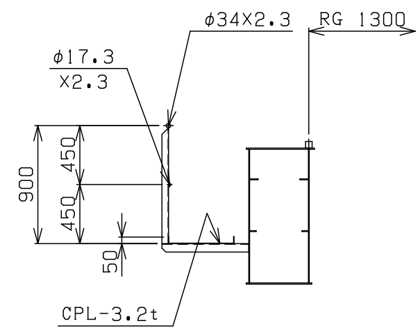
ガーダー断面
